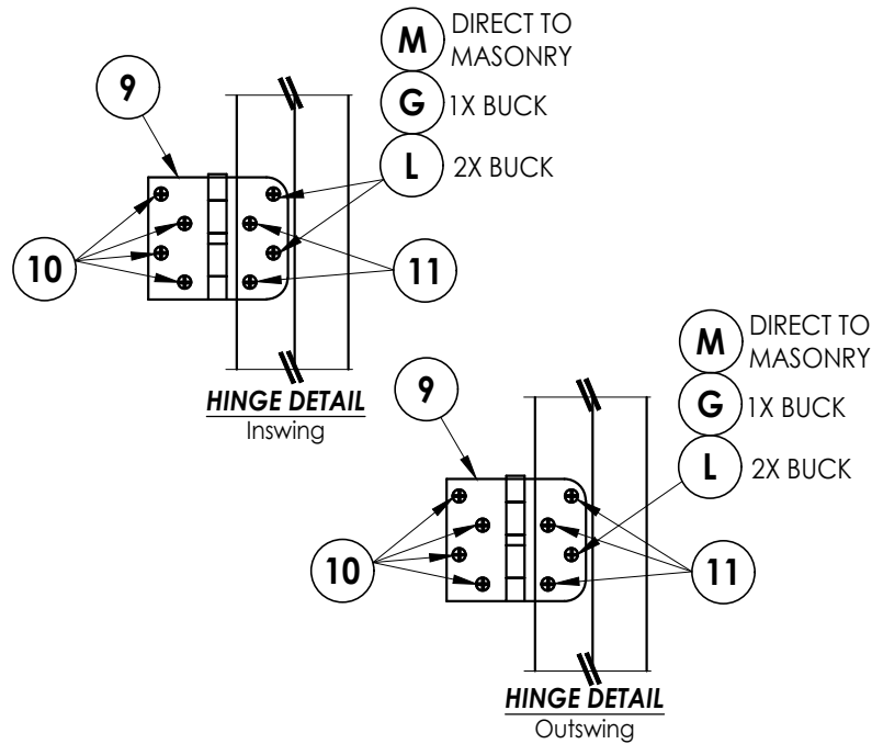
HINGE JAMB
