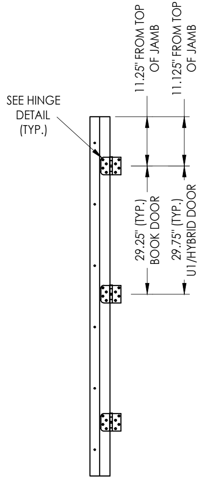
HINGE JAMB
